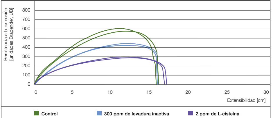
Figura 2: extensograma de masa de harina de trigo preparada con y sin ablandadores de la masa
